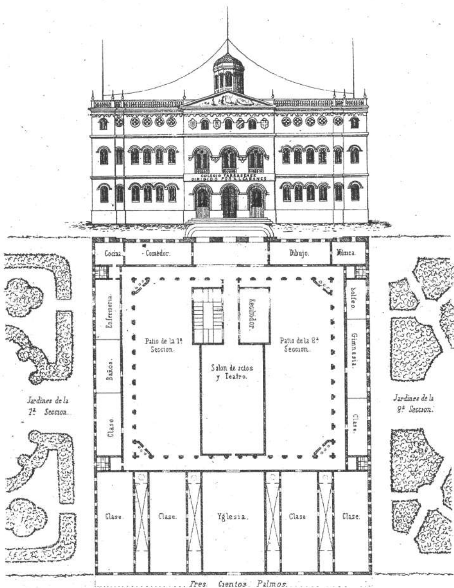
Façana i plànol del Colegio Tarrasense, imprès en paper, de 34 x 25 cm. Arquitecte: Francesc Daniel Molina i Casamajó, maig de 1864. Al frontispici de la façana apareix el nom d'Anselm Cabanes i Prunés en qualitat de director. AHCT
